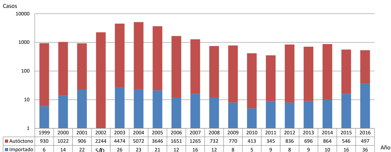
Casos de paludismo según origen, República de Panamá 1999-2016 (sem40)
