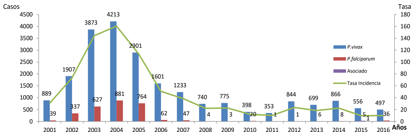
Casos detectados y tasa de incidencia de paludismo según Plasmodium en Panamá 2001-2016 sem 40
